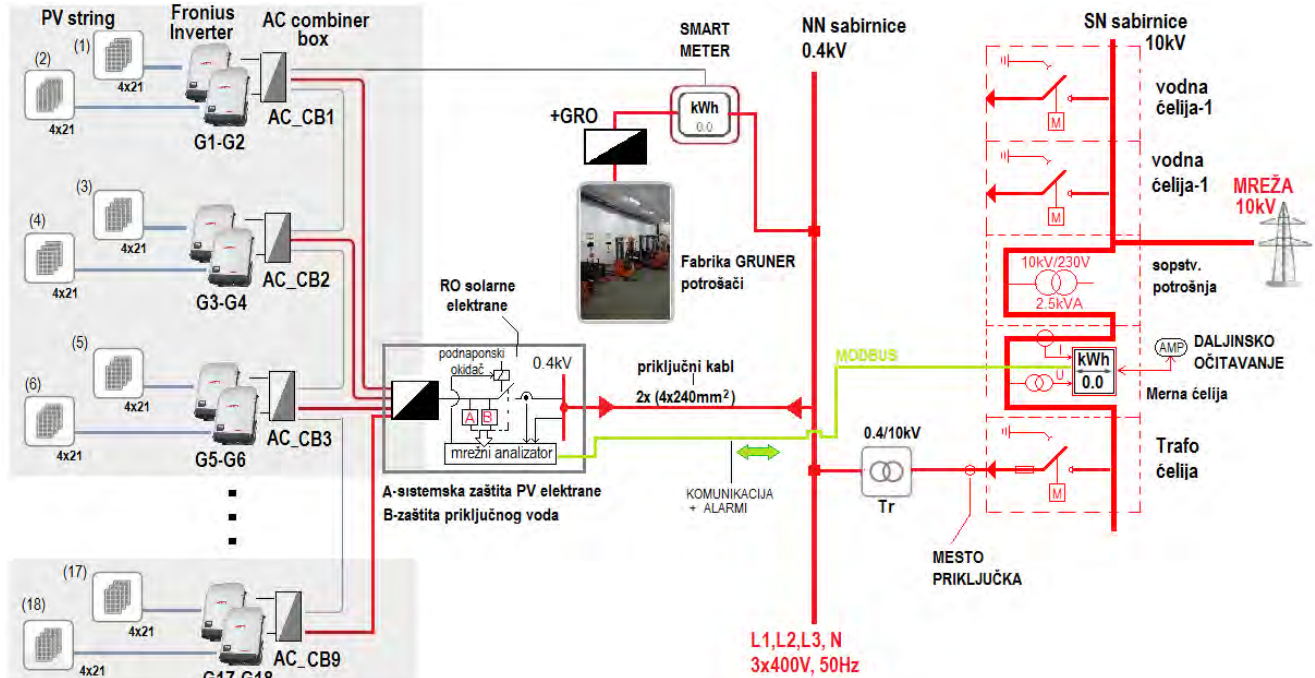
Slika 6. Principalska blok šema fotonaponske elektrane „GRUNER“
