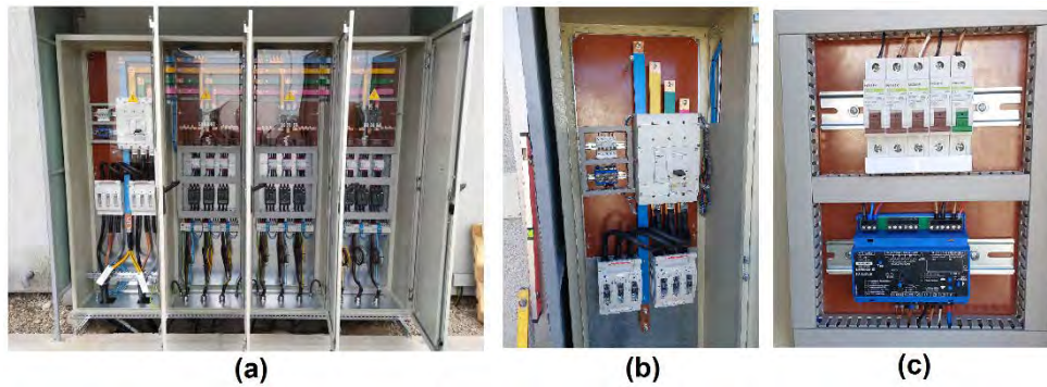
Slika 17. Dispozicija GRO solarne elektrane na naponskom nivou 0.4kW
